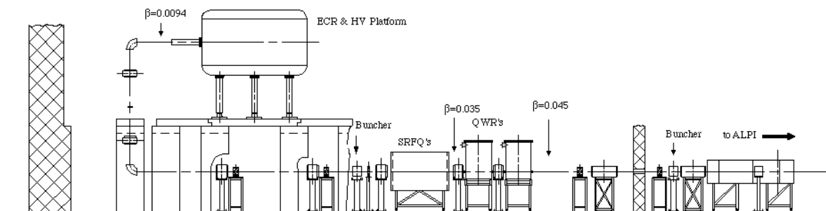
Fig. 1. The PIAVE layout
