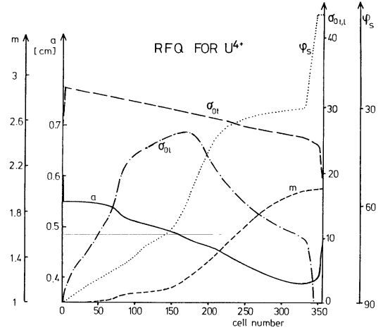
Fig. 3 RFQ parameters for the HSI-RFQ.
